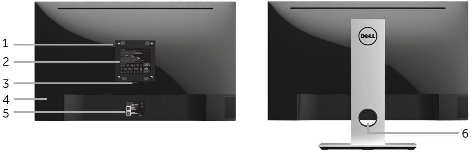
后视图（包括显示器支架）
